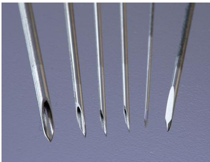
Nadeln elektropoliert / entgratet Material AISI 304
